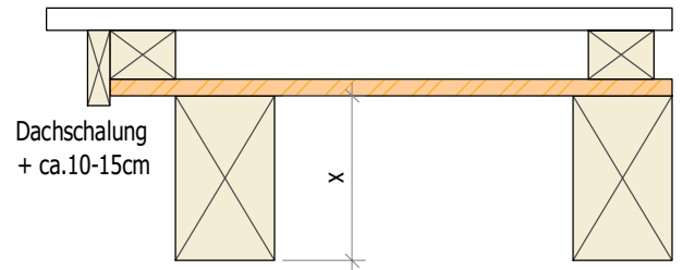
Ortgangdetail ohne Dämmung
