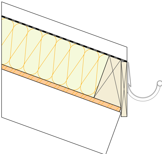
Traufdetail Aufdachdämmung
